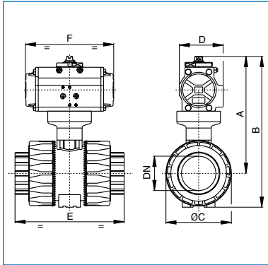
VALVOLA CON ATTUATORE SEMPLICE EFFETTO
