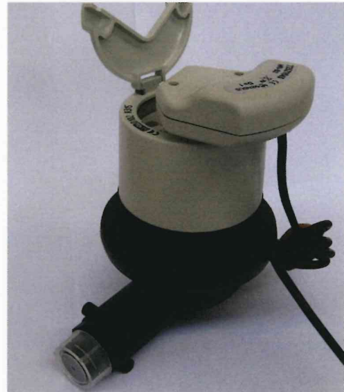
620C Q 3 2,5 mit Kunststoff, gekapseltes Zählwerk (Perspektivdarstellung)
