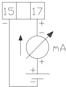
Uscita in corrente passiva
